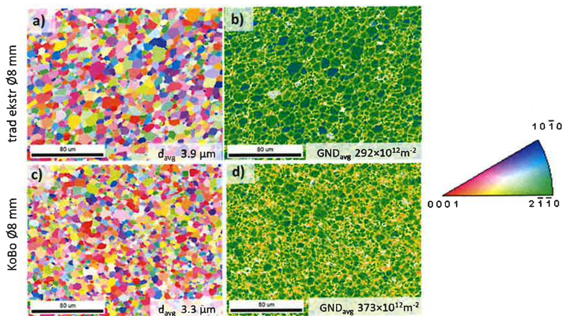
Rysunek 14. Wyniki EBSD dla stopu WE43: a) mapa rozkładu orientacji ziaren stopu odkształconego tradycyjną ekstruzją na gorąco R_1 5:1, b) rozkład dyslokacji geometrycznie niezbędnych (GND) w stopie odkształconym tradycyjną ekstruzją na gorąco R_1 5:1, c) mapa rozkładu orientacji ziaren stopu odkształconego metodą KoBo bez nagrzewania materiału wsadowego R_1 5:1, d) rozkład dyslokacji geometrycznie niezbędnych (GND) w stopie odkształconym metodą KoBo bez nagrzewania materiału wsadowego R_1 5:1 [A6]
