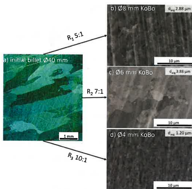
Rysunek 6. Mikrostruktura czystego odlewane Mg oraz czystego Mg po przeróbce metodą KoBo w pojedynczym cyklu przejścia przez zespół matryc bez wstępnego nagrzewania wsadu [A1] przy zastosowaniu różnych stopni odkształcenia: a) materiał wsadowy (odlew), b) R_1 5:1, c) R_2 7:1 oraz c) R_3 10:1
