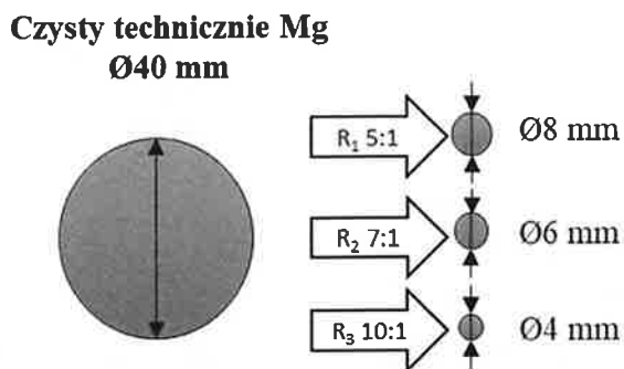
Rysunek 5. Stopnie odkształcenia ( R ) zastosowane dla czystego technicznie Mg przerobionego metodą KoBo bez wstępnego nagrzewania wsadu [A1]
