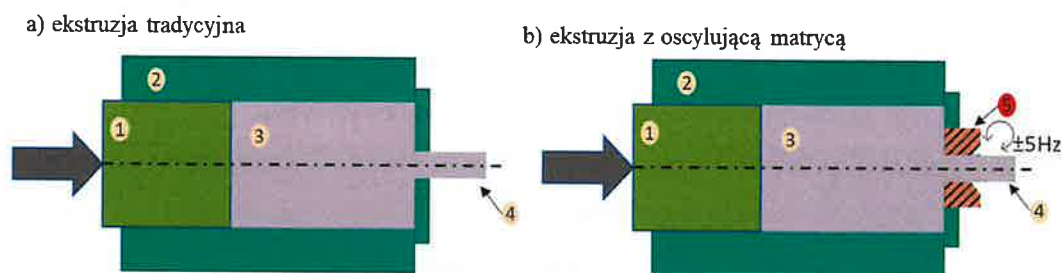
Rysunek 1. Porównanie schematów metod wyciskania: a) tradycyjnego, b) z oscylującą matrycą (1- stempel 2 – tuleja ekstrudera, 3 – materiał przeciskany, 4 – materiał przeciśnięty, 5 – oscylująca matryca) [A6]
