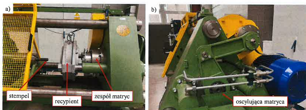
Rysunek 2. Prasa hydrauliczna Hydromet do wyciskania z oscylującą matrycą (metoda KoBo): a) widok układu wytłaczania ze stemplem, tuleją recypienta \varnothing 40 \times 160 mm wraz z zespołem matryc, b) widok z przodu: układ oscylującej matrycy o częstotliwości od 1 Hz do 10 Hz i amplitudzie kąta skrętu od 2^\circ do 12^\circ
