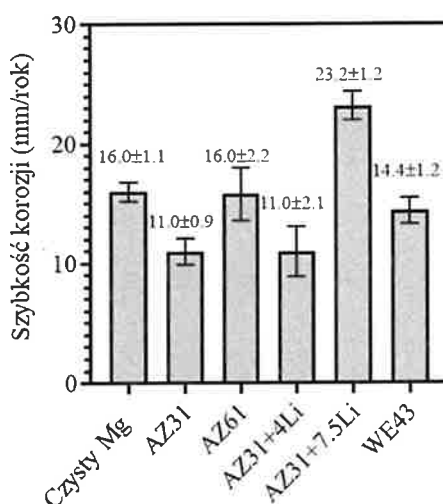
Rysunek 17. Szybkość korozji Mg i jego stopów odkształconych metodą KoBo bez wstępnego nagrzewania wsadu obliczona na podstawie wydzielonego wodoru w roztworze zawierającym jony chlorkowe [A7]
