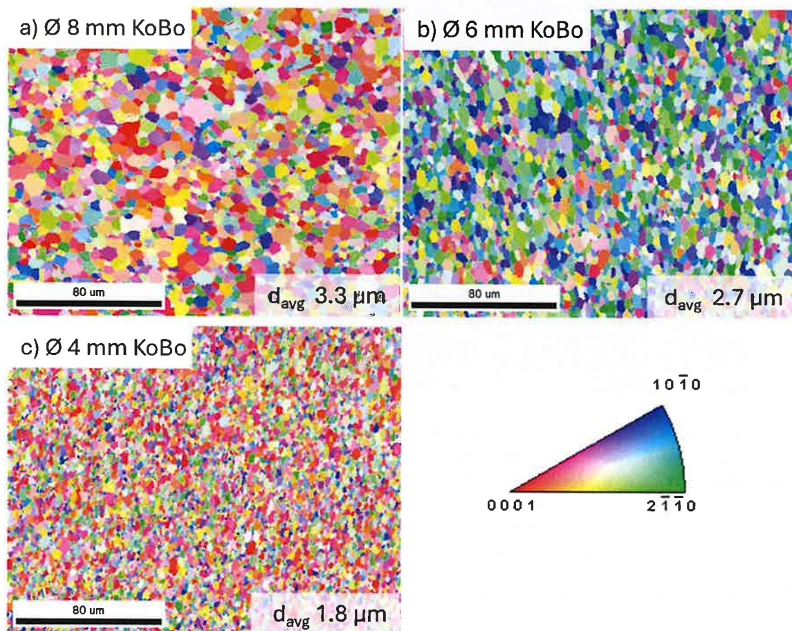
Rysunek 15. Mapy rozkładu orientacji krystalograficznych ziaren dla stopu WE43 odkształconego metodą KoBo bez nagrzewania materiału wsadowego przy różnych stopniach wyciskania: a) R_1 5:1 b) R_2 7:1, c) R_3 10:1 [A6]
